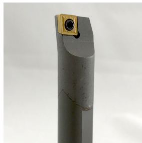
3/8 Ø STUBBY® Carbide Boring Bar C06-SCLCR-2
